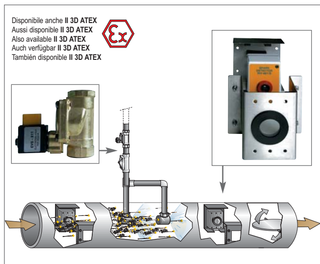
RILEVAMENTO E SPEGNIMENTO SCINTILLA SYSTÈME DE DETECTION ET EXTINGUISHING D'ÉTINCELLES SPARK DETECTION AND EXTINGUISHING SYSTEM FUNKENERKENNUNGS UND FUNKENLÖSCHUNGS SISTEMA DE RELEVADO Y APAGADO DE CHISPAS
